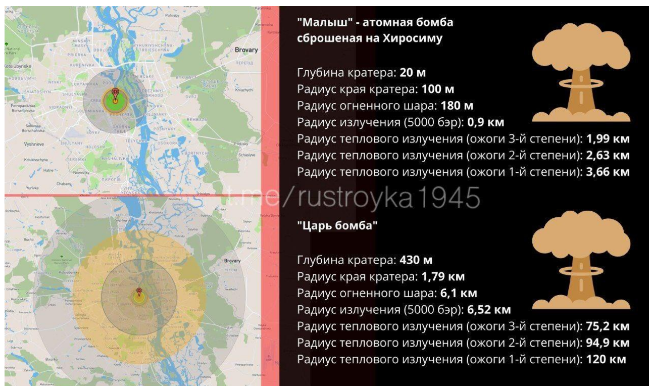
Сравнительная таблица последствий взрыва атомных бомб Хиросимы и советской «Царь-бомбы»
