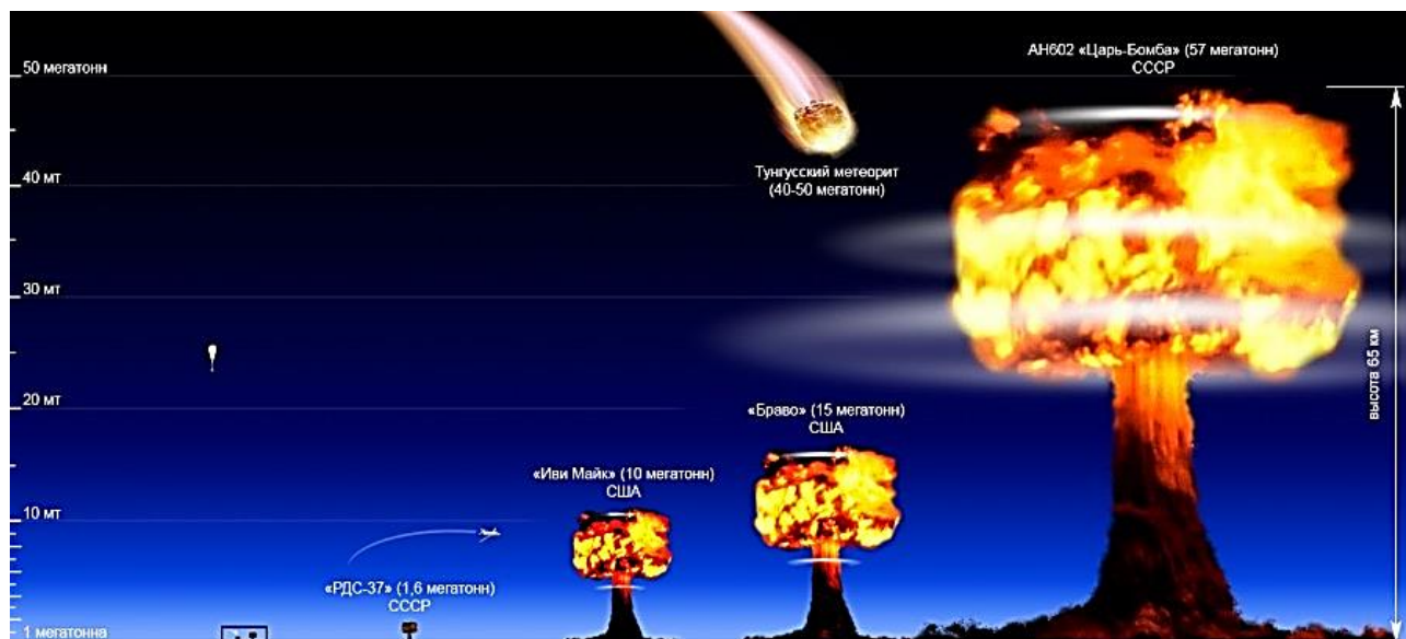
От бомб Хиросимы и Нагасаки (слева в рамочке) – до Царь-бомбы
